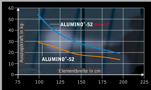
Auszugskräfte aus Standard-Führungsschiene bei Profil ALUMINO 52 protect
