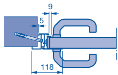
Profiltyp 1 (nur nach innen öffnend)
