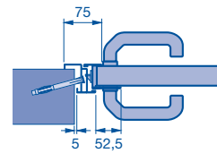
Innenanschlag (nach innen öffnend), Profiltyp 1 oder 2
