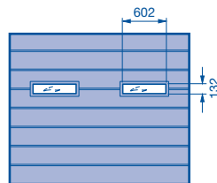
mit Verglasung Typ D
